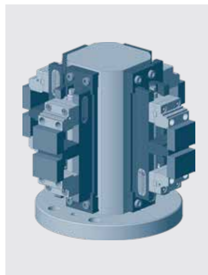
Mechanische Doppelspanner MDU 220-60 auf Spannturm 90° Mechanical double vises MDU 220-60 on a clamping tower 90°
