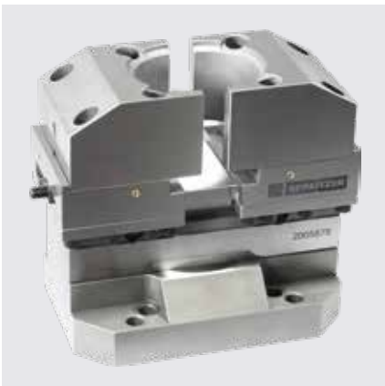
Hydraulischer Zentrischspanner HZS 180-80 A mit Sonderspannbacken Hydraulic centre-clamping vise HZS 180-80 A with custom designed jaws
