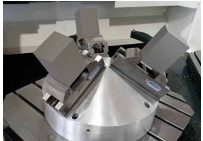
Drei mechanischer Zentrischspanner MZR auf einer Pyramide Three mechanical centre-clamping vises MZR on a pyramid
