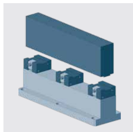
Drei Rohteilspanner RS in Reihe Three raw part clamping units RS in line
