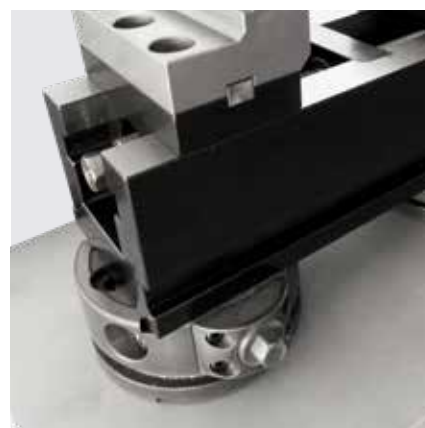
Zentralspanner MZU auf Spanneinheit ZPS mit Indexierung Centre-clamping vise MZU on clamping unit ZPS with indexing
