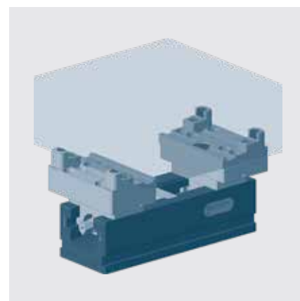
Mechanischer Zentrischspanner MZU 360-125, Pendelbacken mit Gripeinsätzen KG 2 Mechanical centre-clamping vise MZU 360-125, pendulum jaws with grip inserts KG 2
