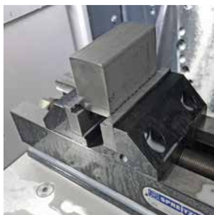
Mechanischer Zentrischspanner MZE 220-80 mit Gripbacken Mechanical centre-clamping vise MZE 220-80 with grip jaws
