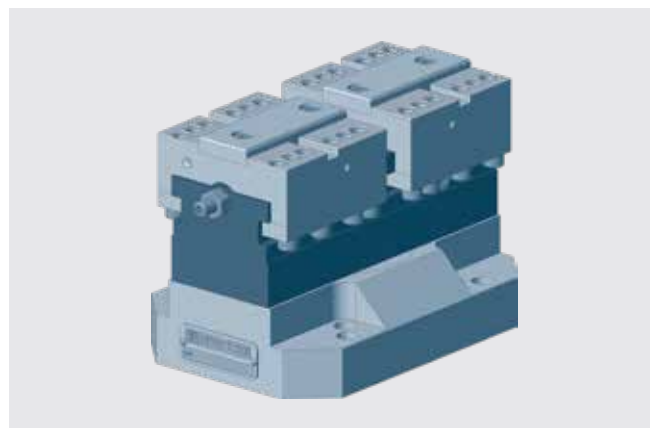
Hydraulischer Zentrischspanner HZS2 180-80, Spannbackenschnittstelle mit Spitzverzahnung Hydraulic centre-clamping vise HZS2 180-80, clamping jaw connection by fine serration
