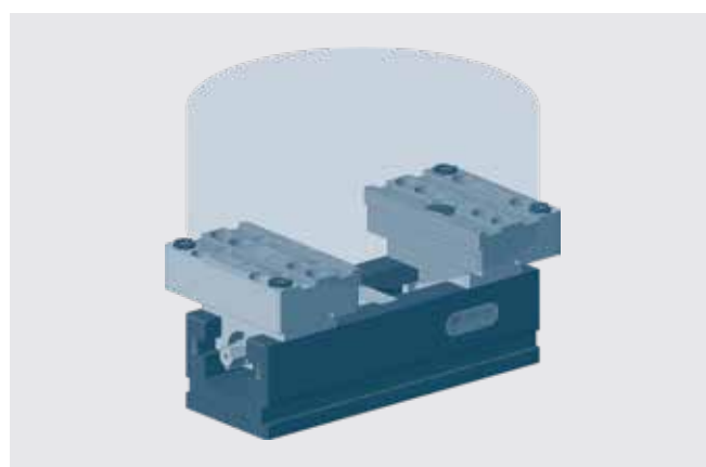
Mechanischer Zentrischspanner MZU 360-125, Pendelbacken mit Gripeinsätzen ZG Mechanical centre-clamping vise MZU 360-125, pendulum jaws with grip inserts ZG
