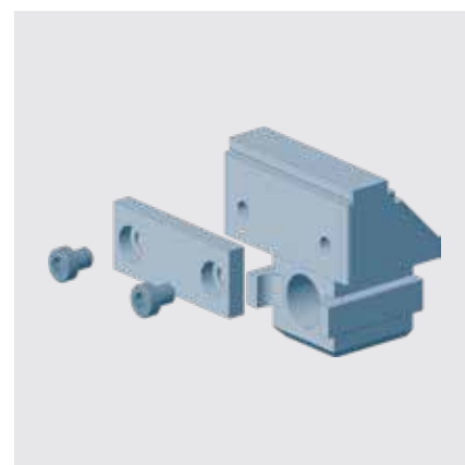
Wendebacken, glatt mit Auflageleiste auf Anfrage Reversible jaws, flat with support rail upon request
