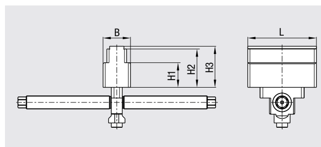
Maße MZE / MZU Dimensions MZE / MZU
